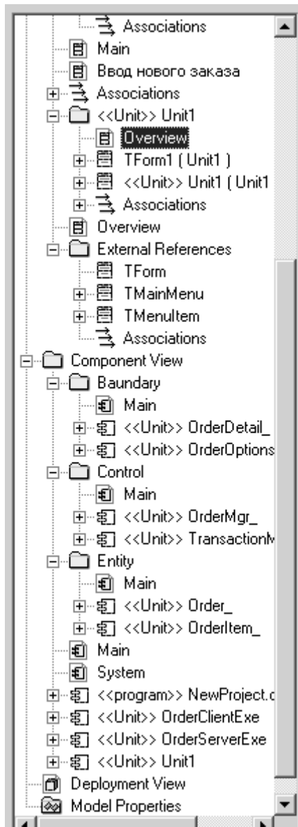
Рис. 16. Окно Rose Delphi Link после кодогенерации
