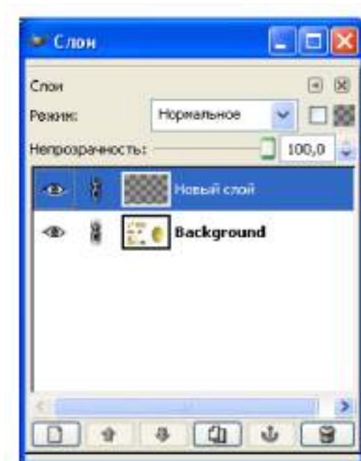
Рисунок 16 - Диалог слоев
